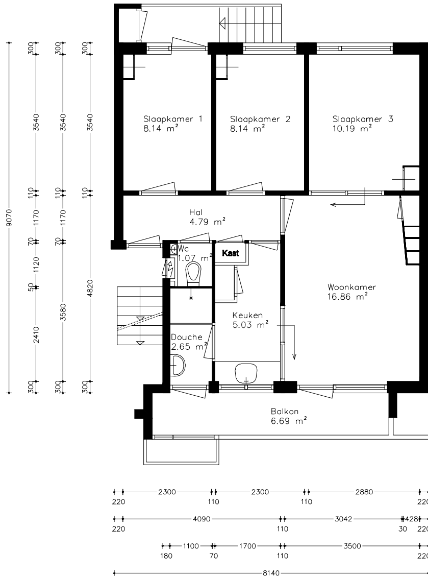
Begane grond
